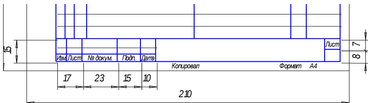
Рисунок 5.4 – Основная надпись для спецификаций (последующие листы)
